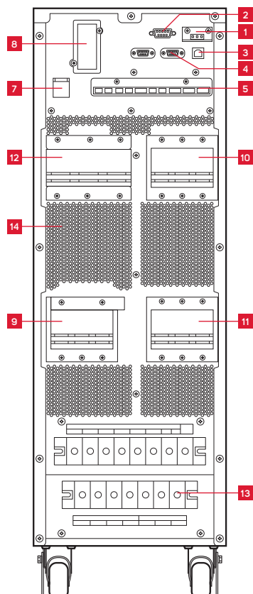
HE3340XL (40 кВА / 36 кВт)
