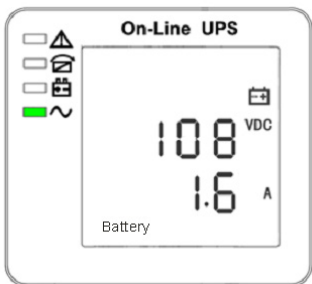
(4) Напряжение и ток АКБ+ (положительная группа) (5) Напряжение и ток АКБ- (отрицательная группа)
