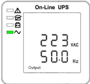
(3) Выходные параметры
